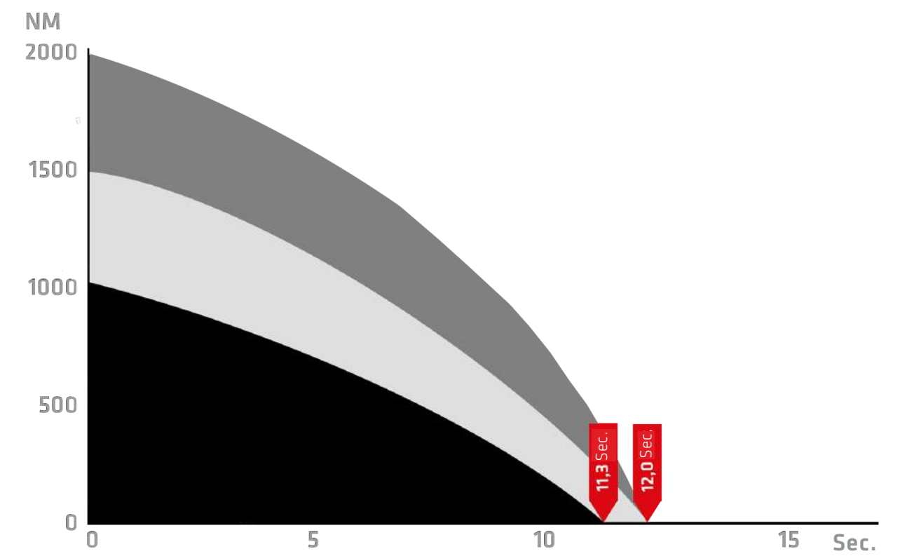
Kihajtás: Nyomaték görbék összehasonlítása
