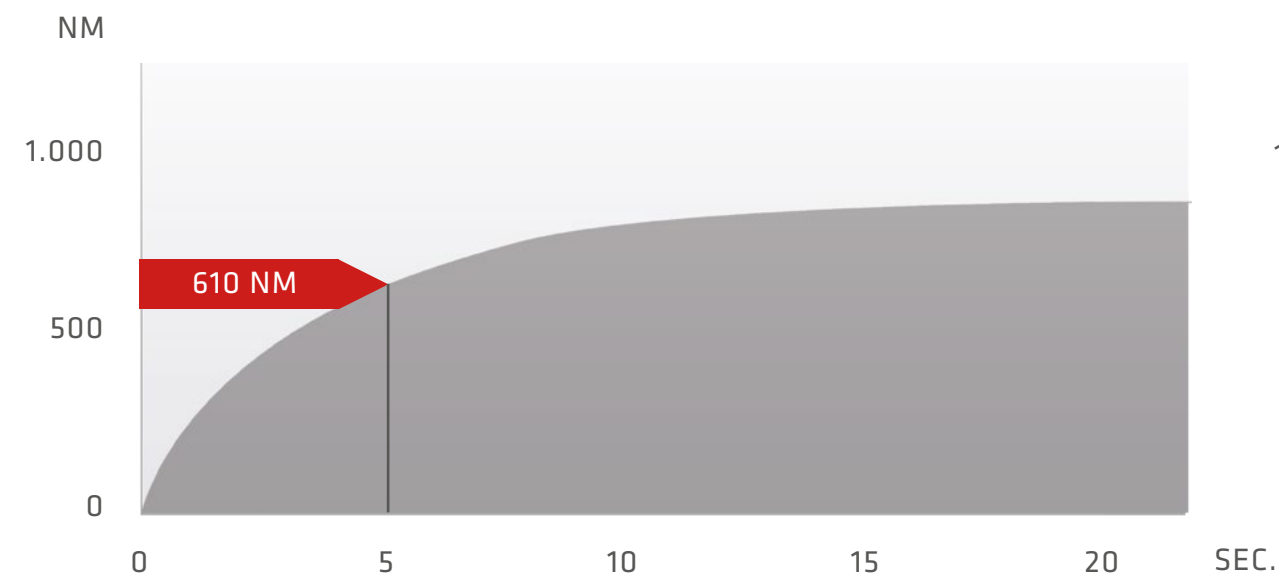
Meghúzás (behajtás 2): az SW C5144 nyomaték görbe
